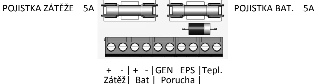
Obrázek 4 – Označení svorek
