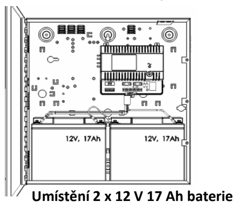
Obrázek 2 – Umístění baterií - kryt velikosti „E“
