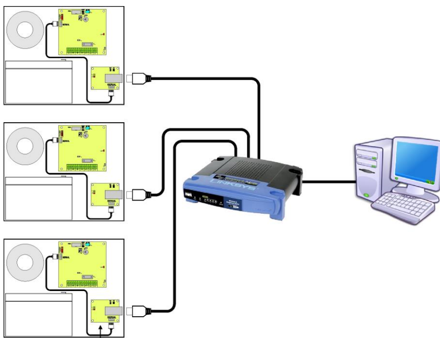
Obr. 12. Komunikace přes síť Ethernet s použitím rozhraní „INTE”.
