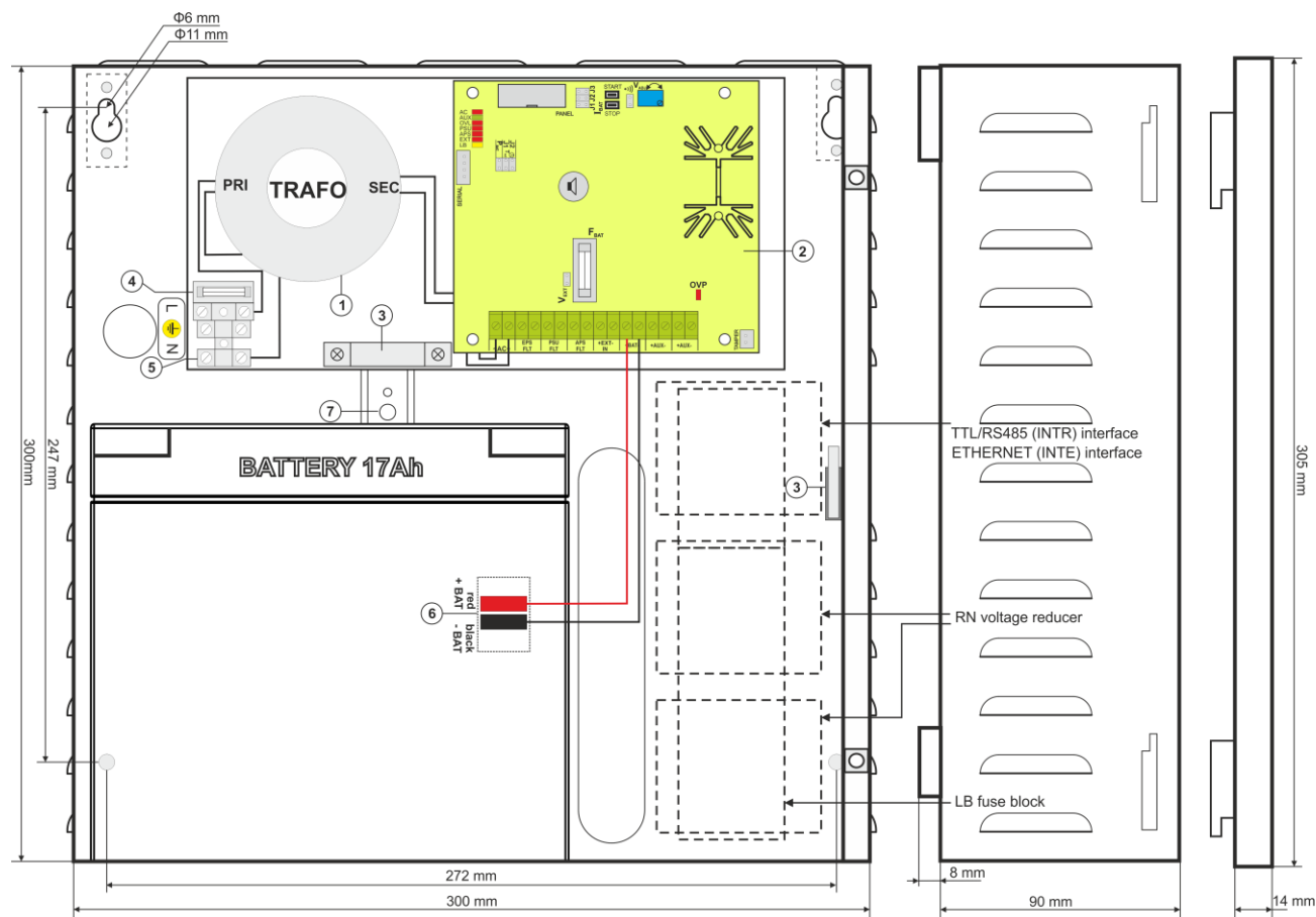
Obr.3. Zobrazení PSU.
