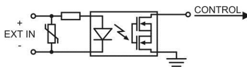
Obr. 9. Elektrické schéma vstupu EXT IN.
