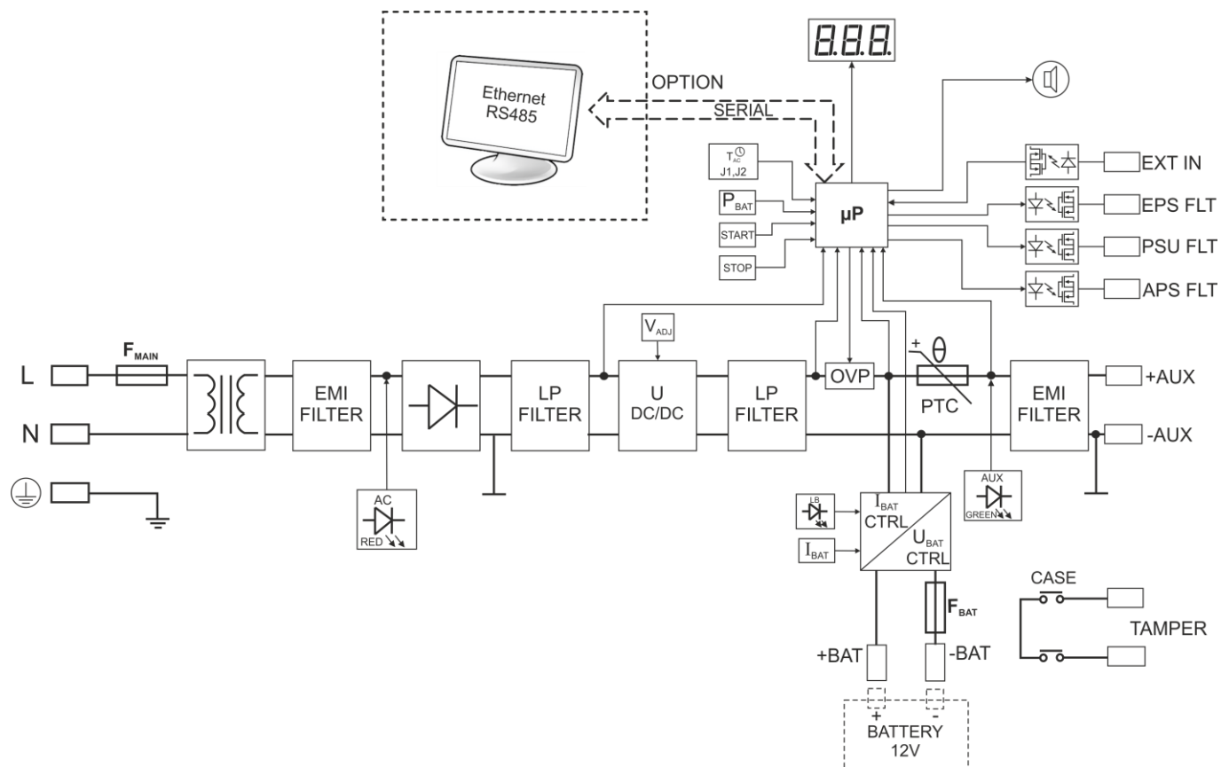
Obr. 1. Blokové schéma PSU.
