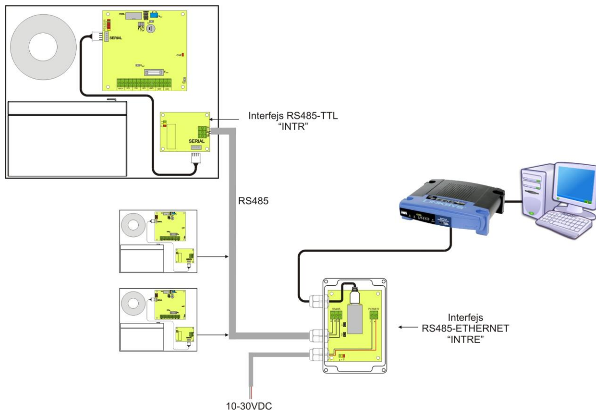
Obr. 13. Komunikace přes síť Ethernet s použitím rozhraní RS485-Ethernet „INTRE”.
